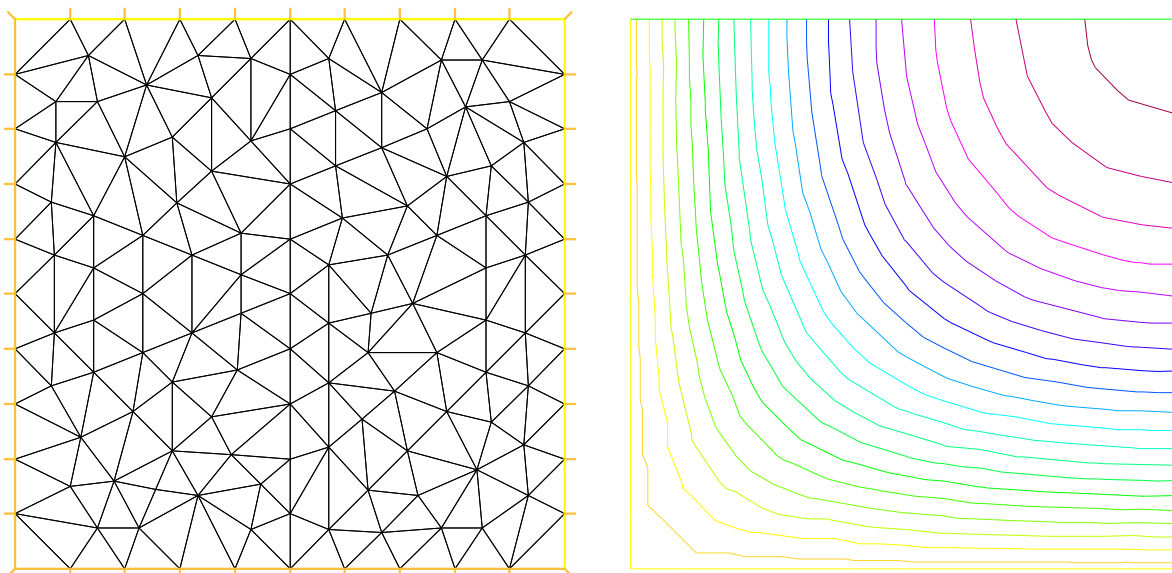
図 5: poisson-kikuchi.edp — 要素分割と解の等高線
