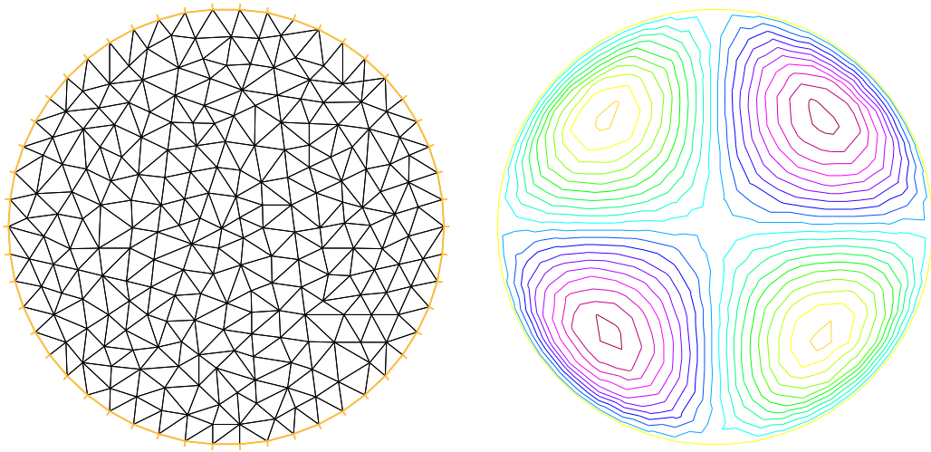
図 2: 円盤領域で Poisson 方程式 -\Delta u(x, y) = xy の同次 Dirichlet 問題を解く (三角形要素分割と解の等高線)
