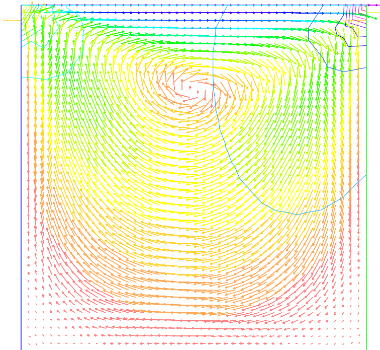
図 10: P2/P1 (分割は粗くした)
