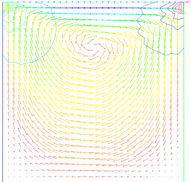
図 8: stokes-p1b.edp の結果
