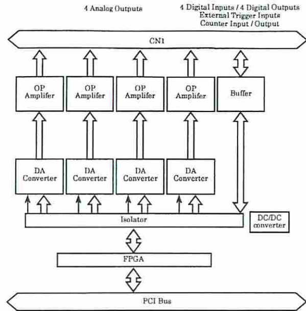
図6.3 回路ブロック図<DAI16-4(LPCI)L>
