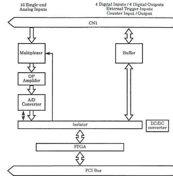
図6.2 回路ブロック図<ADI16-16(LPCI)L>
