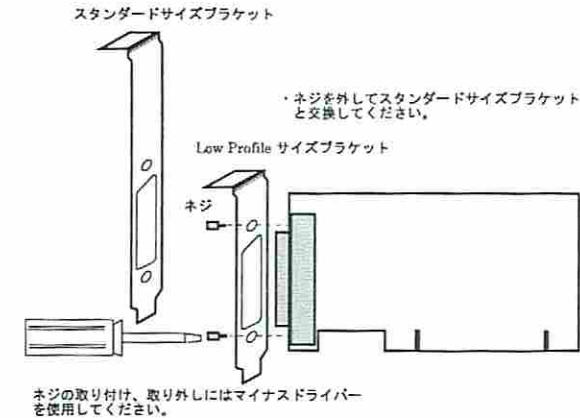
図2.1 ブラケットの交換
