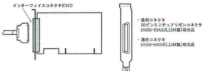
図3.1 インターフェイスコネクタの形状
