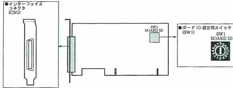
図2.2 各部の名称
