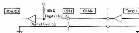
図3.9 デジタル入力の接続
