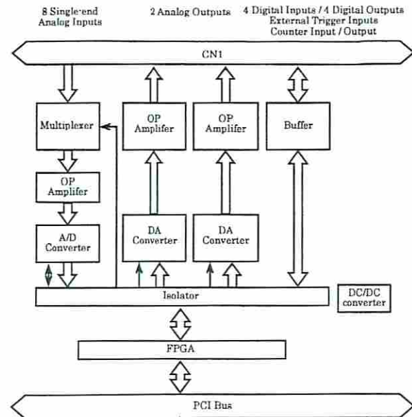
図6.1 回路ブロック図<ADAI16-8/2(LPCI)L>
