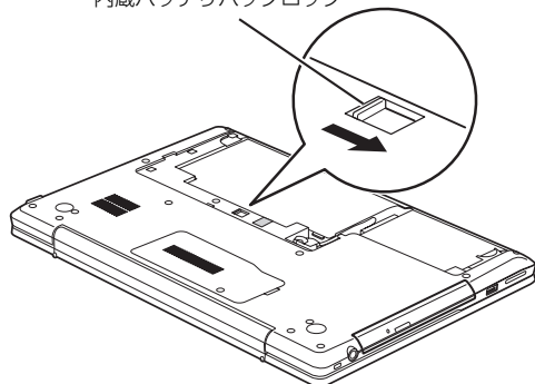
内蔵バッテリーパックロック
