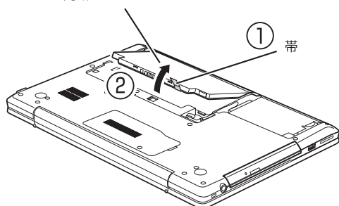
内蔵バッテリーパック
