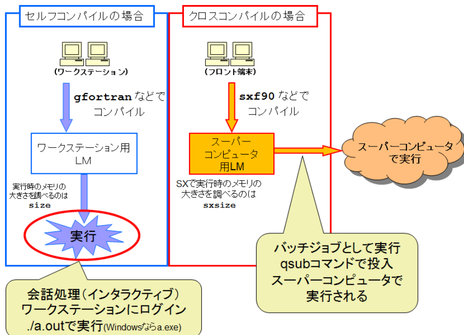
図 14 セルフコンパイラとクロスコンパイラ
