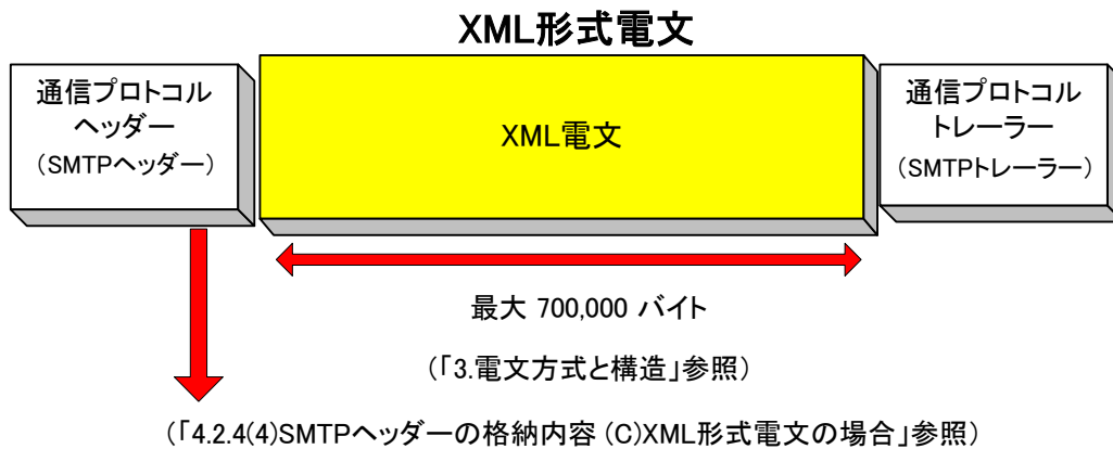
図 4-2-9 XML 形式電文の概要（インタラクティブ処理方式（SMTP 双方向））
