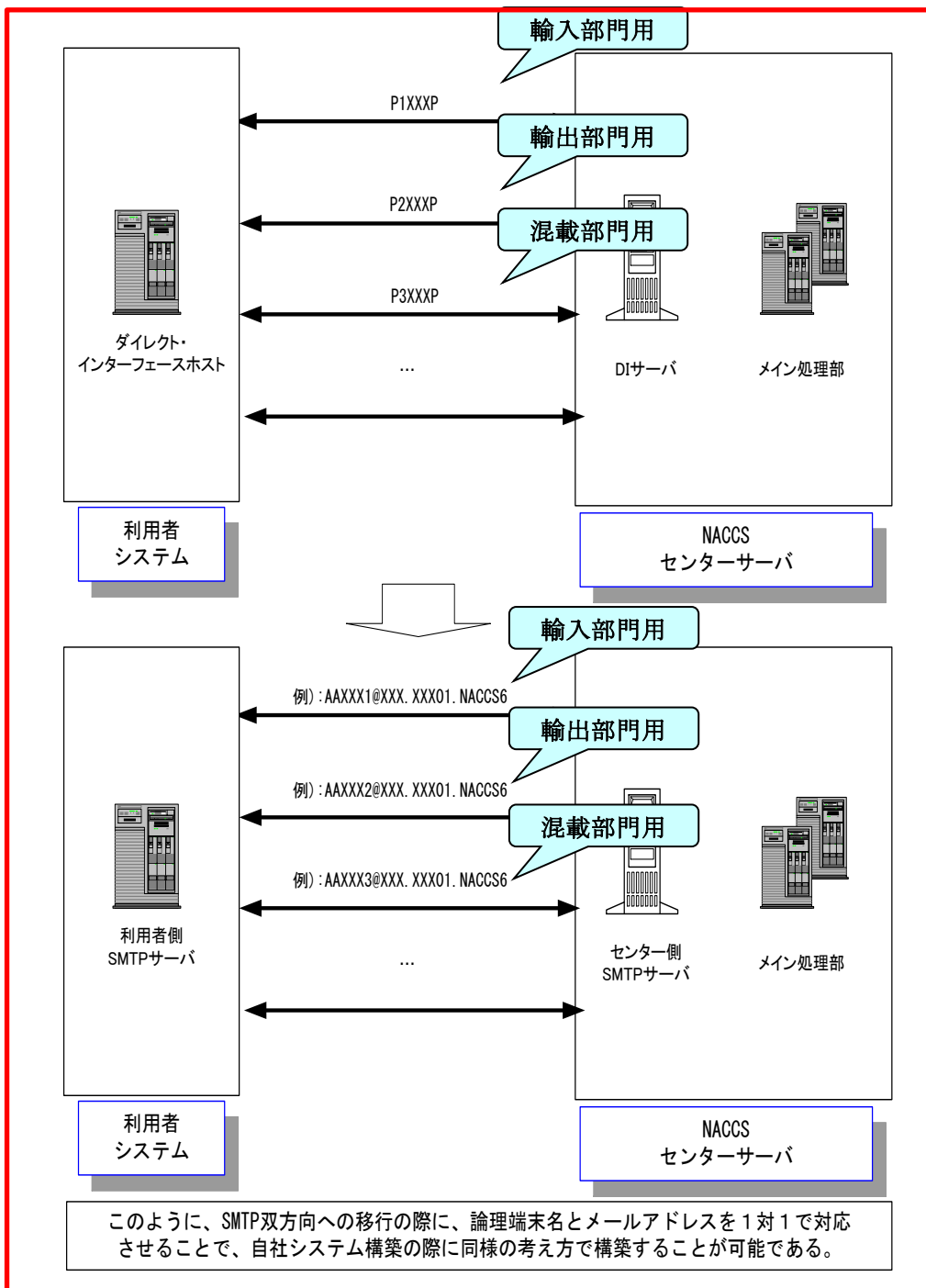
図 4-2-18 【削除】 — インタラクティブ処理方式（ダイレクト・インターフェース）における論理端末名と インタラクティブ処理方式（SMTP双方向）におけるメールアドレスの対応イメージ
