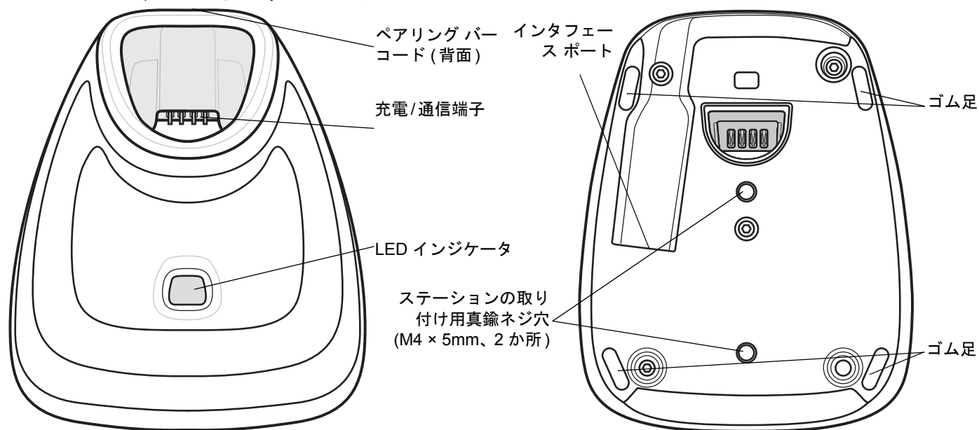
図 1-3 CR2278-PC (プレゼンテーション クレードル) - 上面図と底面図
