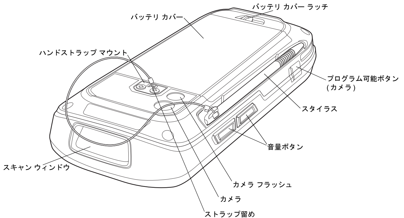
図 1-2 MC45 背面図
