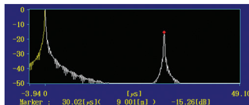
希望波 + 遅延波 の一例 (遅延プロファイル)
