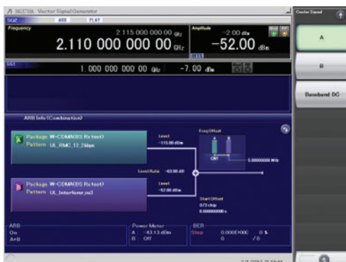
希望波 + 変調妨害波 の設定例
