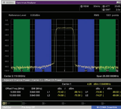
W-CDMA 1キャリアのACLR測定例 (TestModel1, 64DPCH)
