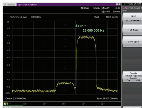
希望波 + 変調妨害波 の一例 (スペクトラム)
