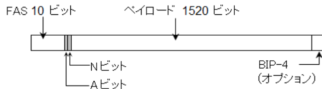
E3 フレーム構造
