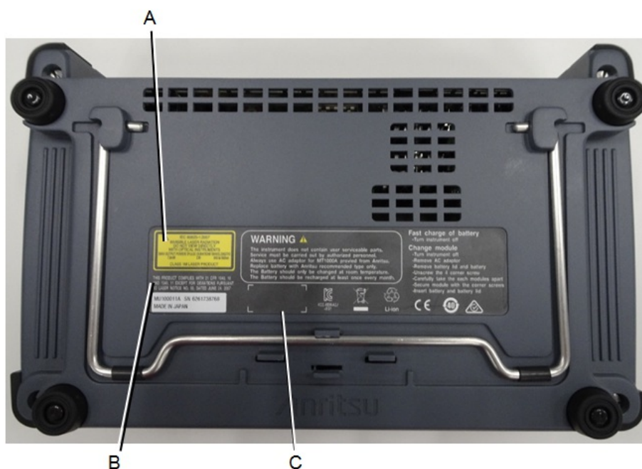
図4 ラベルの貼付位置 (MU100011A)
