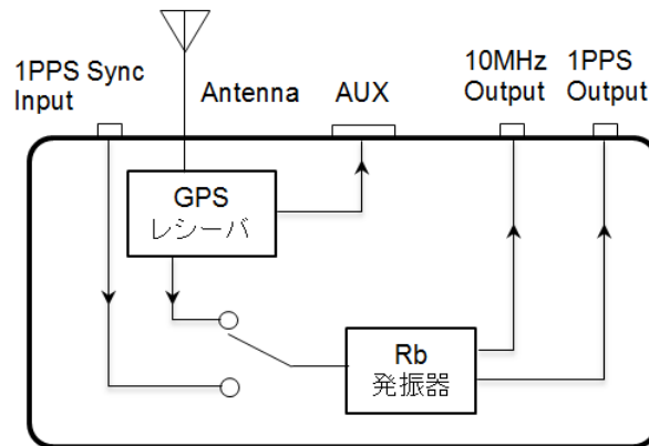
MU100090A ブロック図
