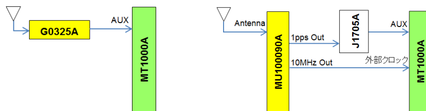
[GPS] 選択時: G0325Aの接続
