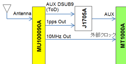
[GPS(外部基準10MHz)] 選択時: MU100090Aの接続
