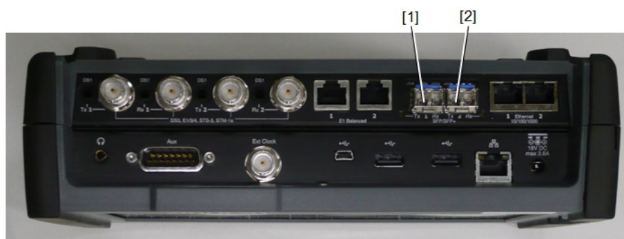
図1 レーザ光の開口位置 (MU100010A)
