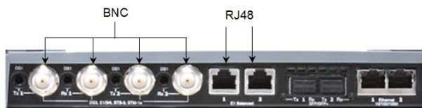
MU100010A コネクタパネル
