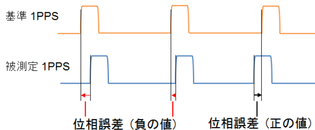
位相誤差の定義
