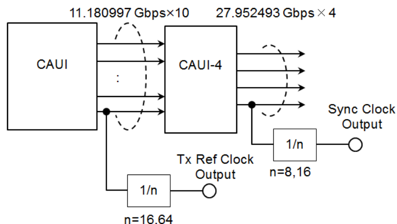
MU100011A 送信部のブロック図
