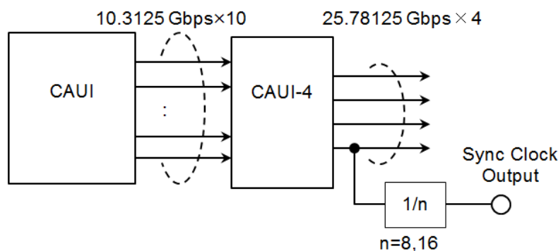
MU100011A 送信部のブロック図 (QSFP28, CFP4)
