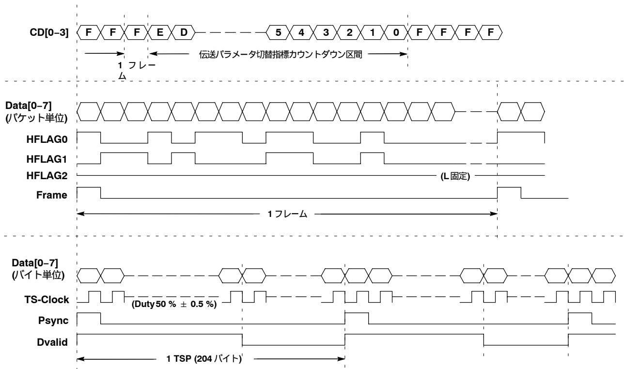
図 E-1 : Universal In/Outコネクタにおける信号間のタイミング関係
