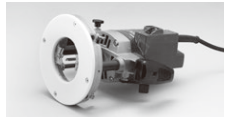
ベースプレートをコーリアン®にしたルーター
