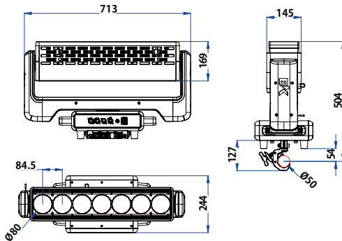
寸法図
