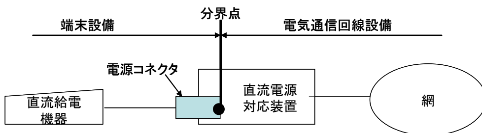
図 2.3-1 直流電源対応装置を利用する場合の分界点
