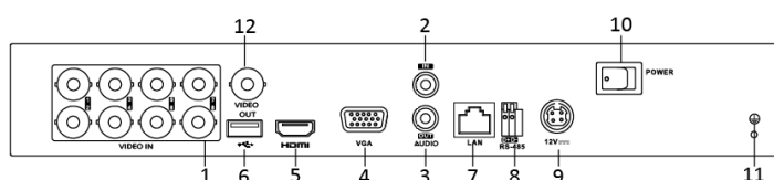
図 1.11DS-7200HQHI-F1/N のリアパネル
