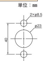
パネルカット図
