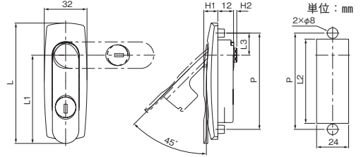
パネルカット図
