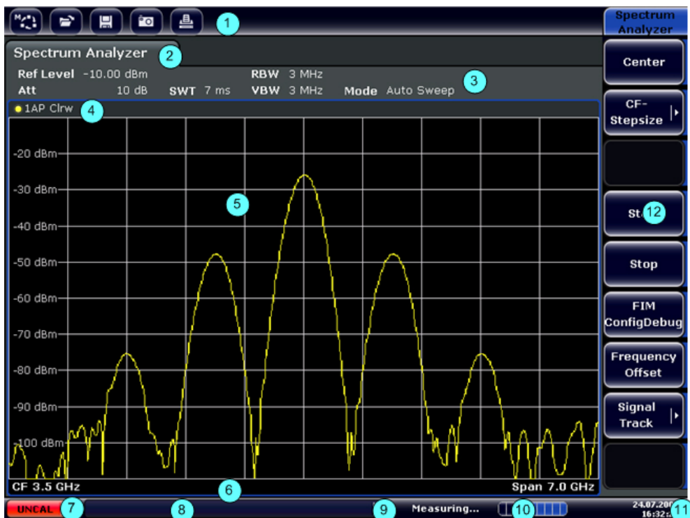
図 5-1: アナライザとして動作中の本機のスクリーン・レイアウト
