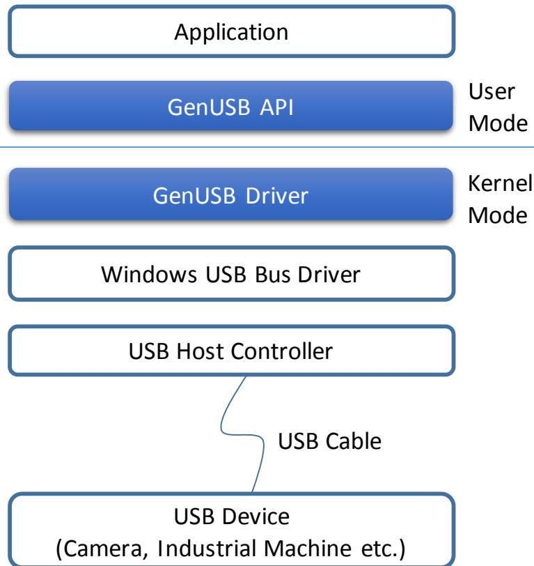
GenUSBドライバ構成図
