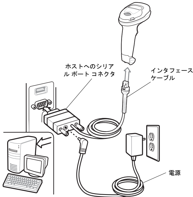
図 8-1 RS-232 接続
