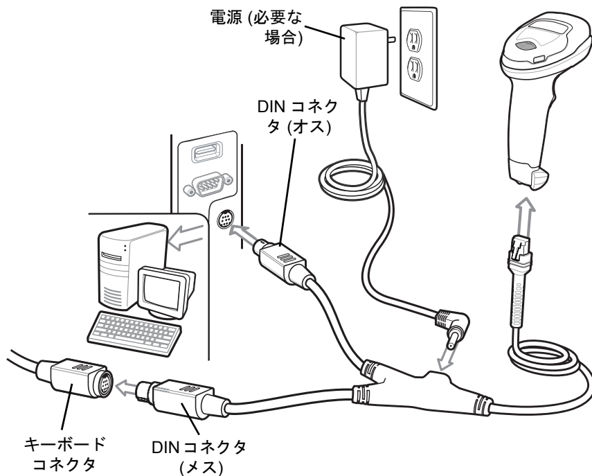
図 10-1 キーボード インタフェースの接続
