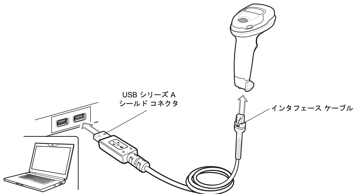
図 6-1 USB 接続
