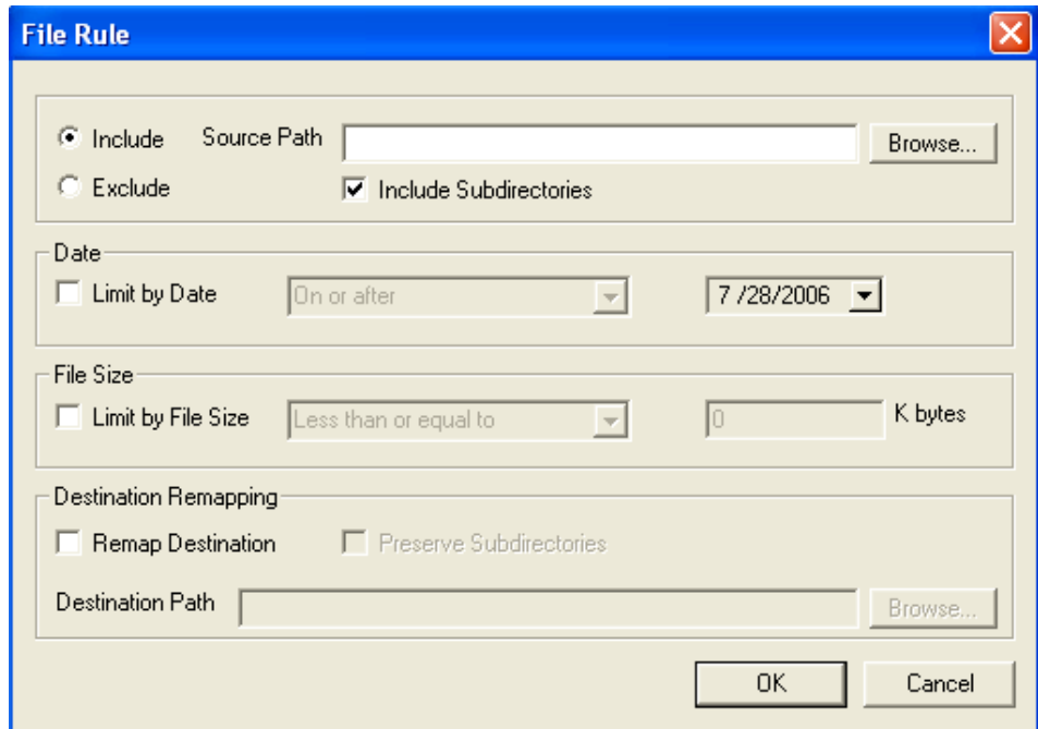
図 39 [File Rules] ダイアログ ボックス
