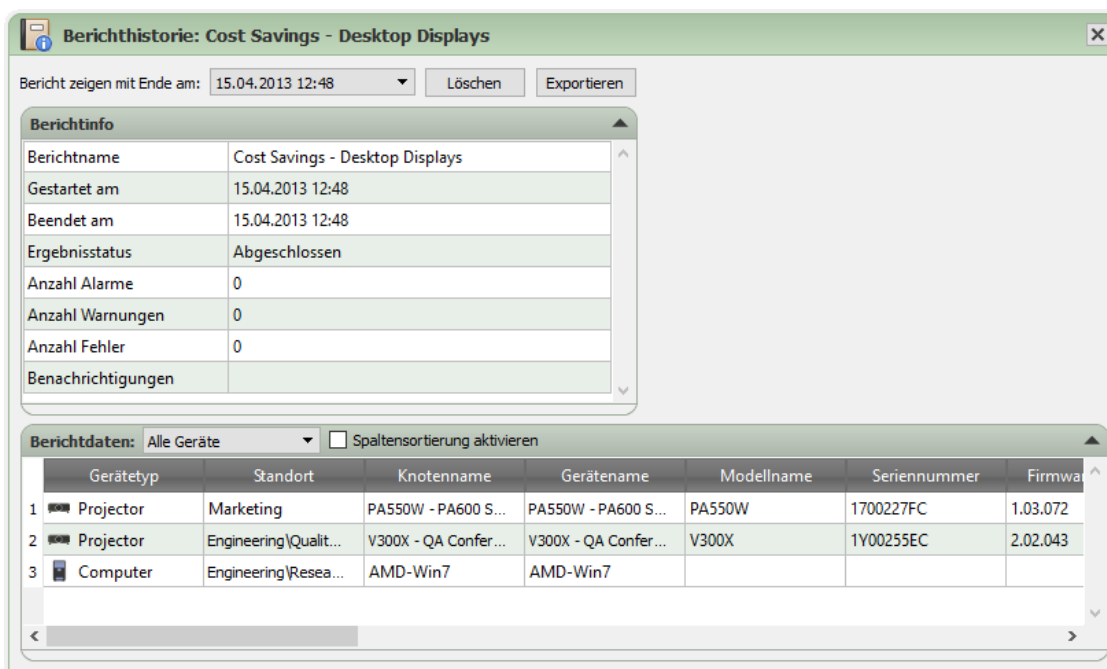
Andockfenster Berichthistorie
