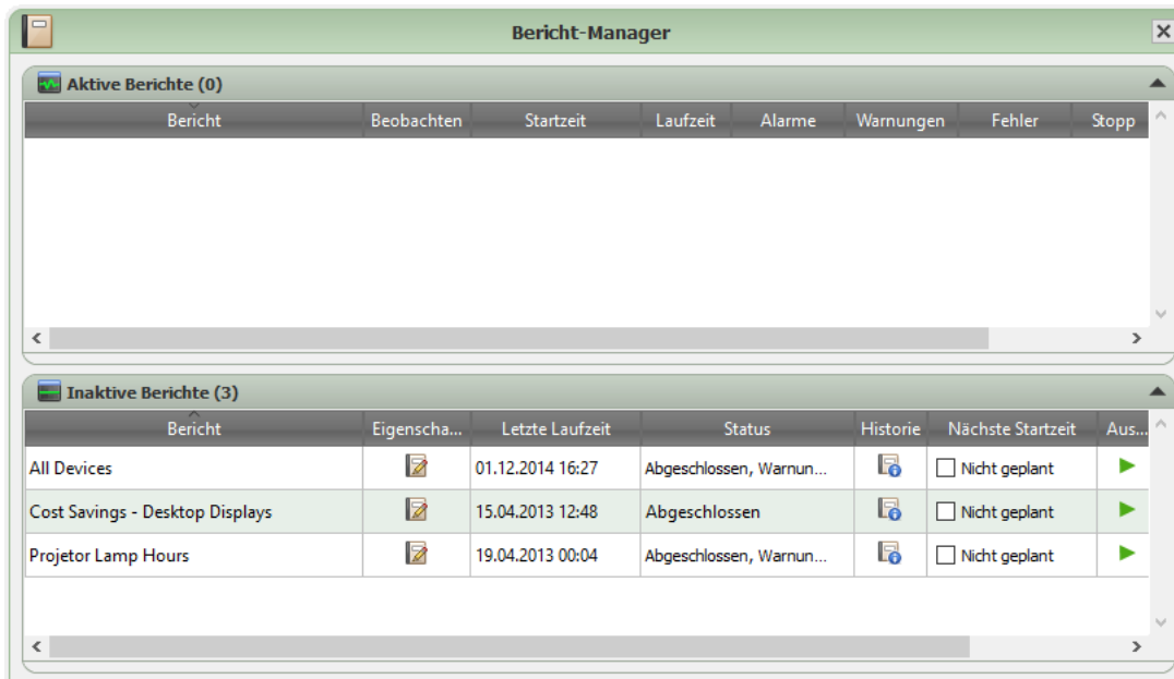
Andockfenster Bericht-Manager
