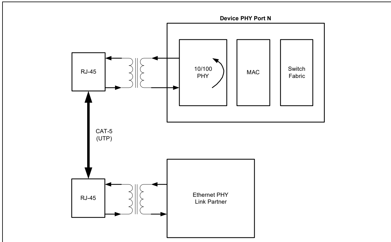
図 4-2: リモート PHY ループバック
