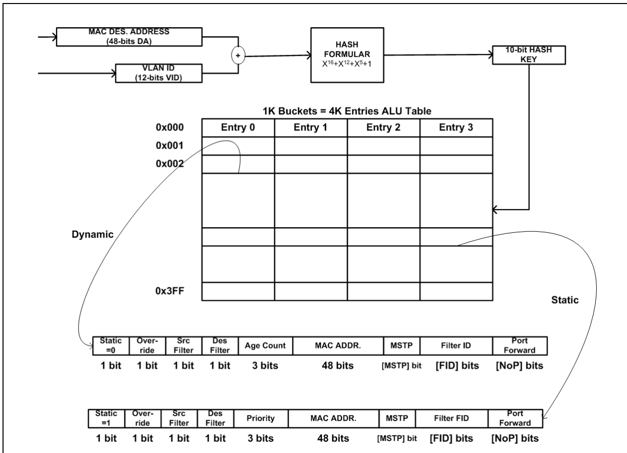
図 5-3: アドレス ルックアップ テーブルの設定
