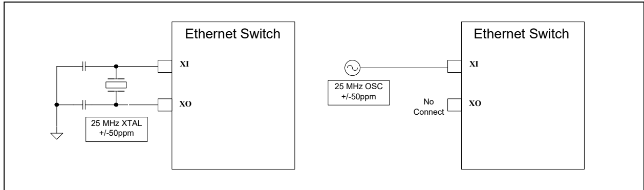
図 6-14: 入力参照クロックの接続方法
