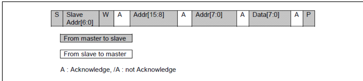
図 4-14: 1 バイトレジスタ読み出し
