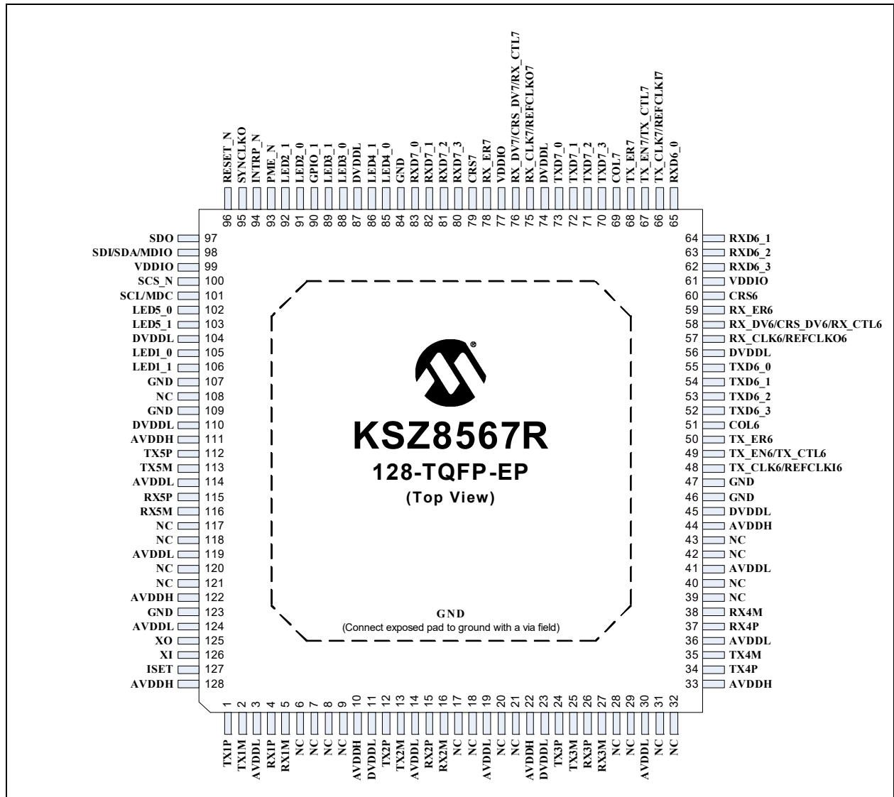
図 3-1: ピン配置図 (上面)
