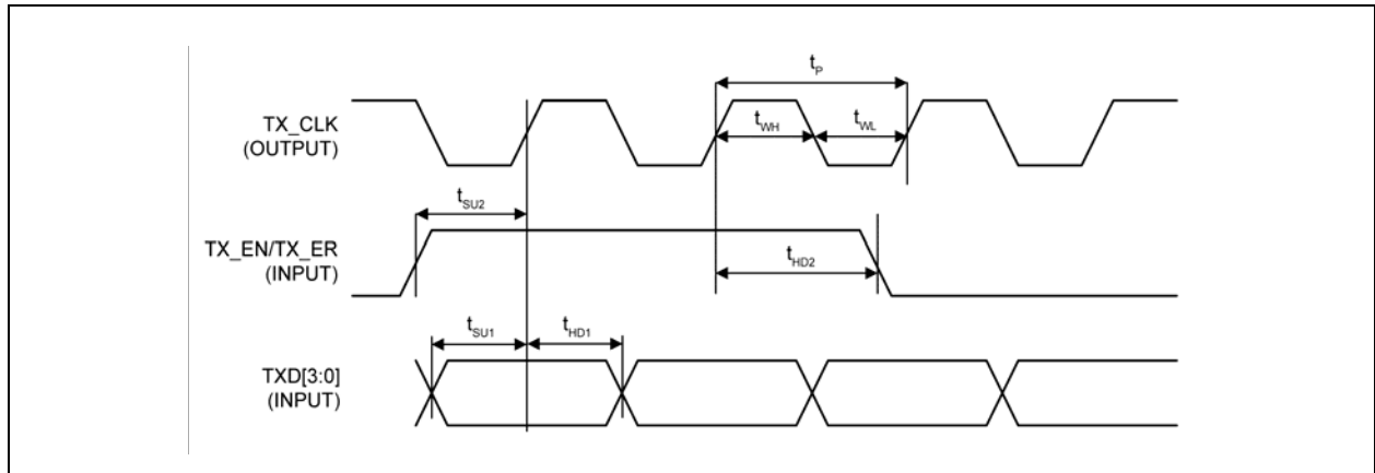
図 6-5: PHY モードの MII 送信タイミング
