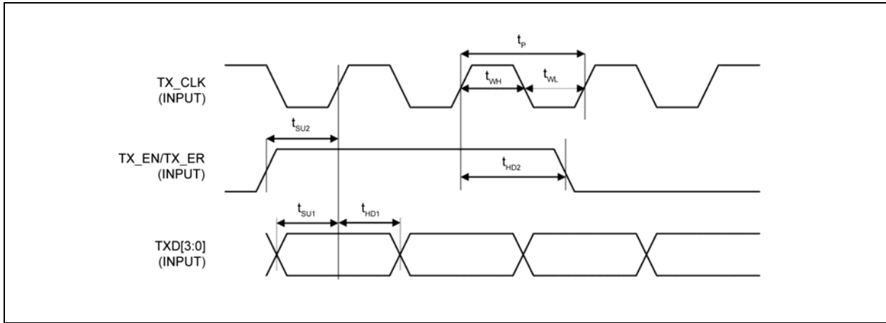
図 6-2: MAC モードの MII 送信タイミング
