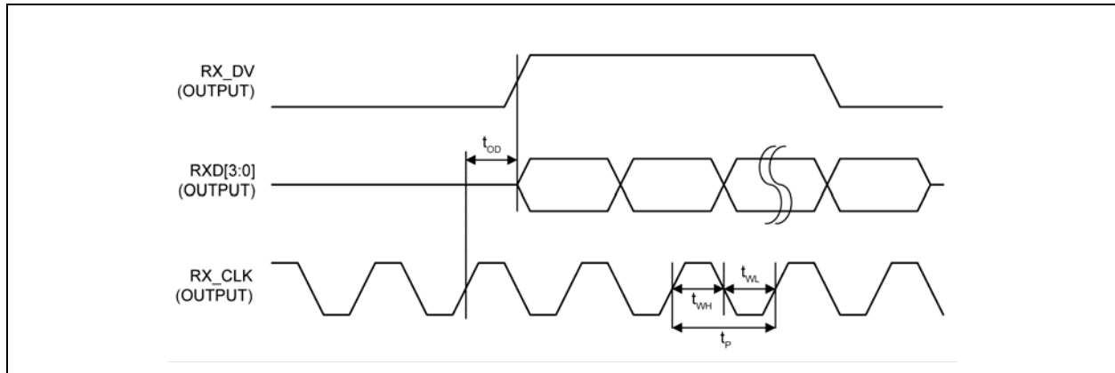
図 6-4: PHY モードの MII 受信タイミング
