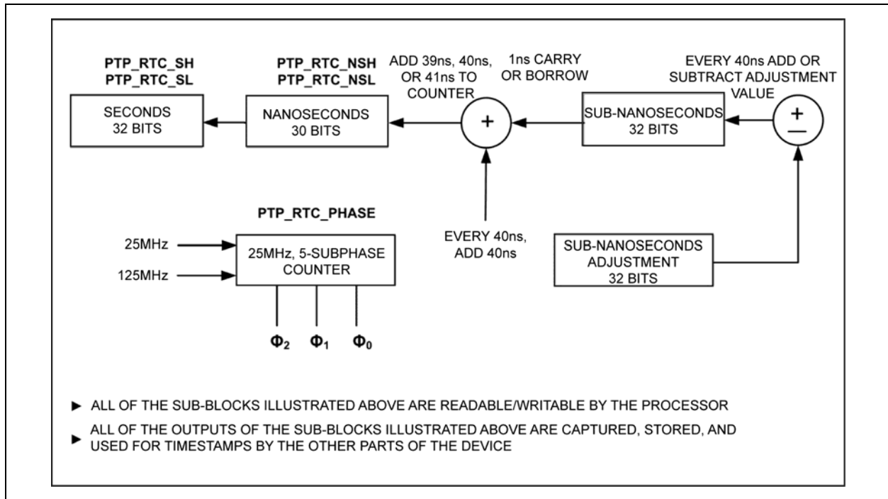
図 4-8: PTP システムクロックの概要
