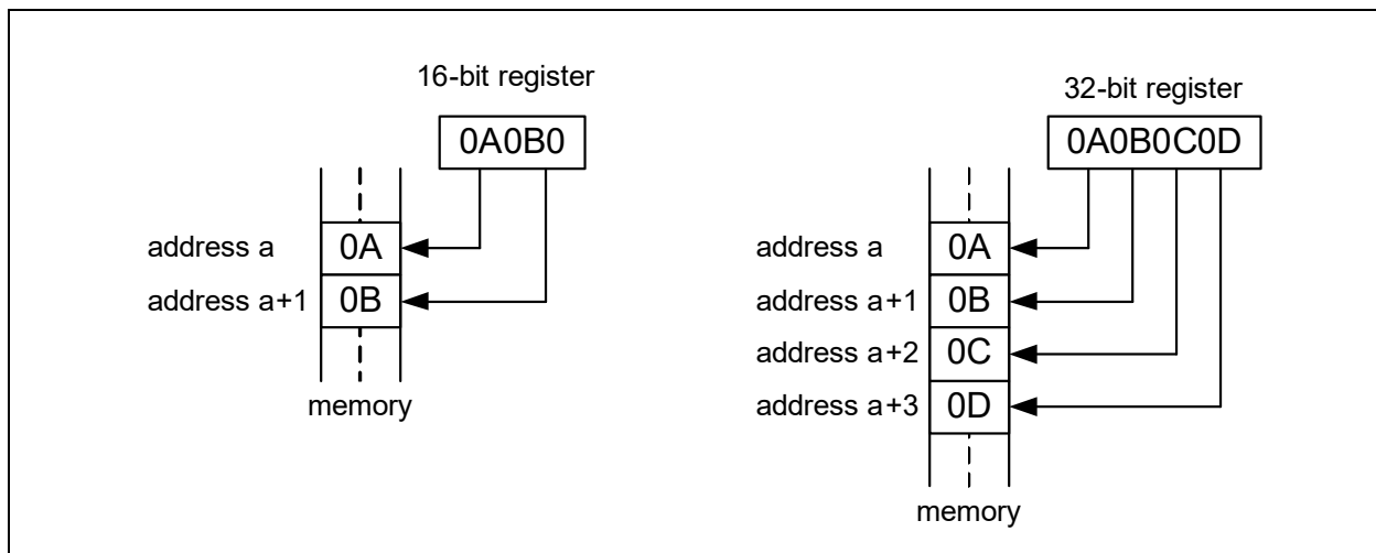
図 5-2: バイトの順序
