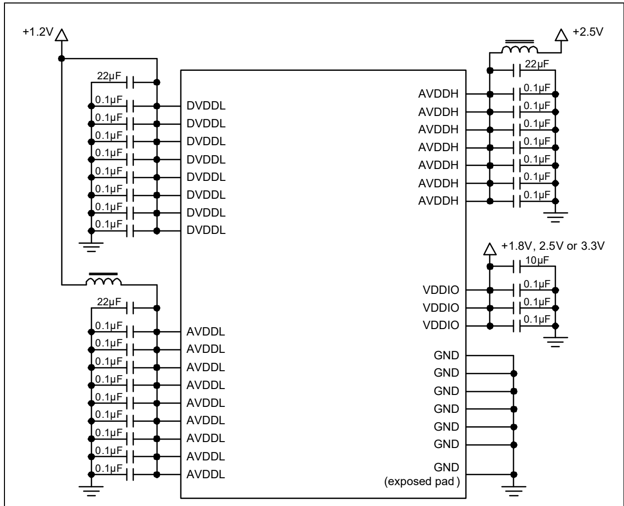
図 4-9: 電源接続図
