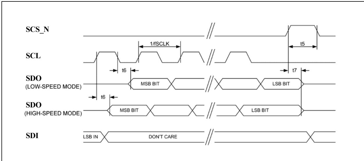
図 6-10: SPI データ出カタイミング
