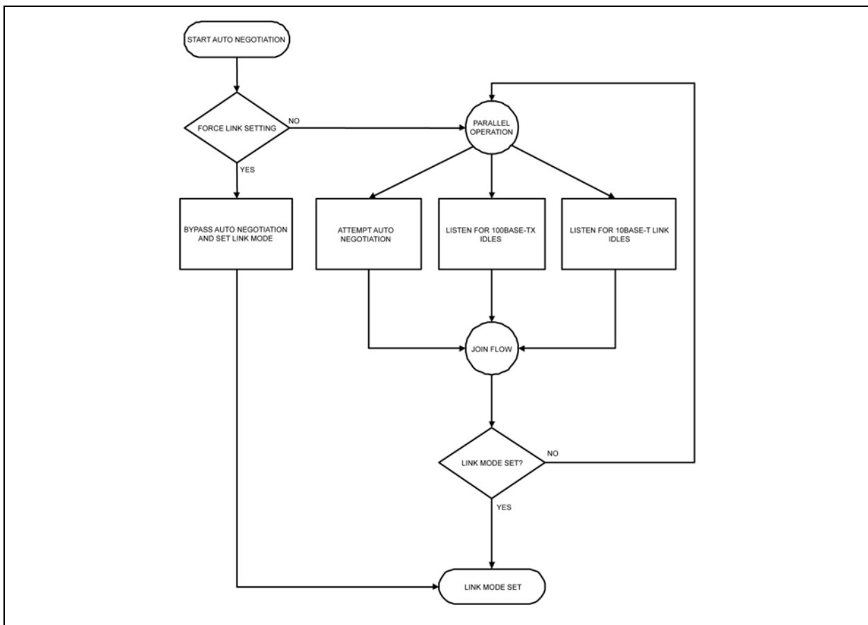
図 4-1: オート ネゴシエーションとパラレル動作
