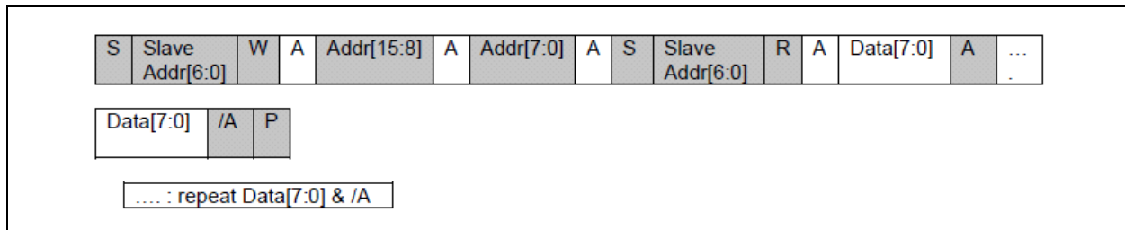
図 4-16: バーストレジスタ読み出し
