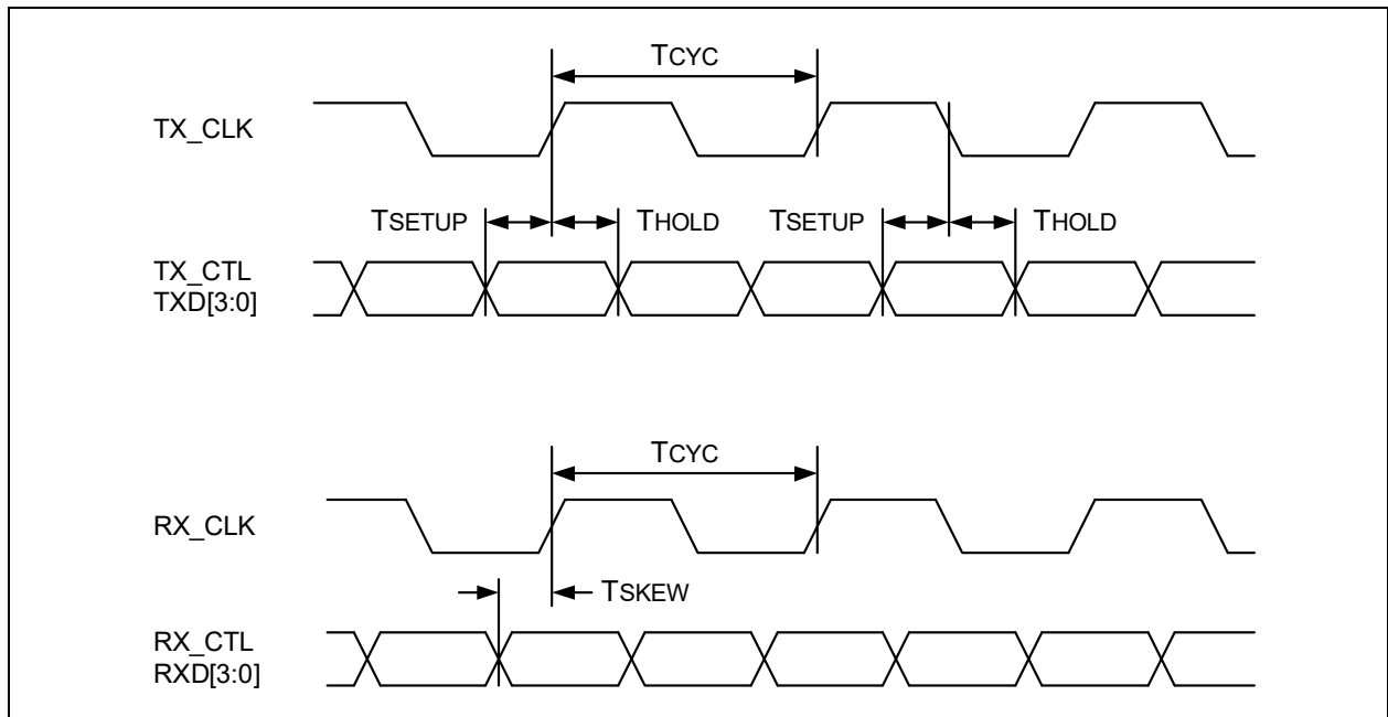
図 6-1: RGMII タイミング
