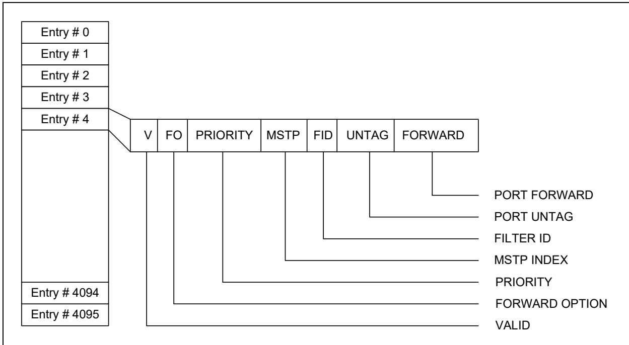
図 5-4: VLAN テーブルの構成
