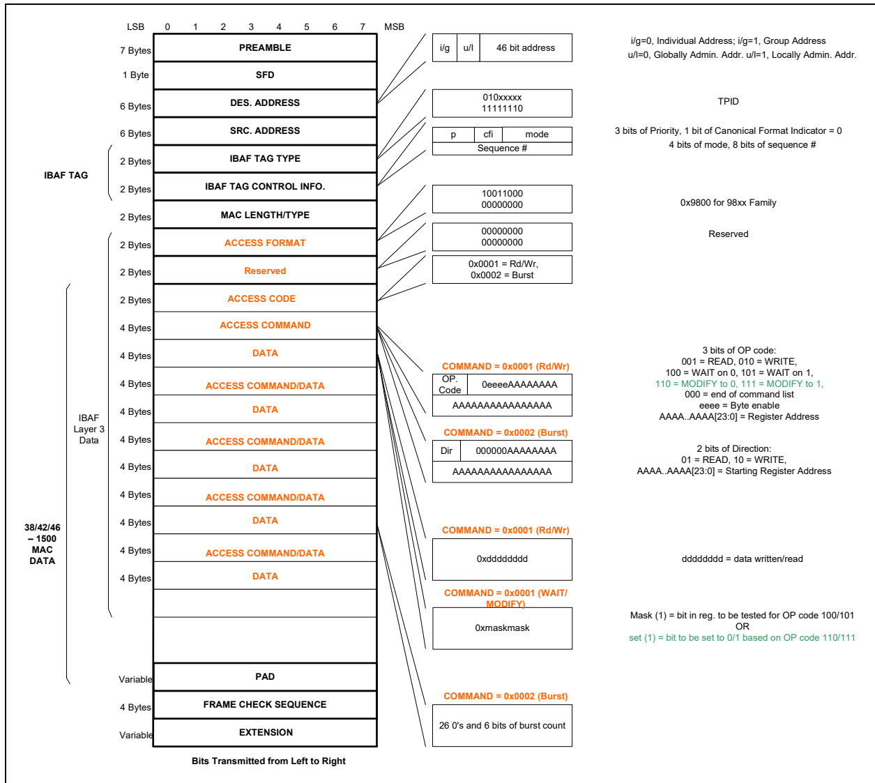
図 4-17: インバンド管理フレームのフォーマット
