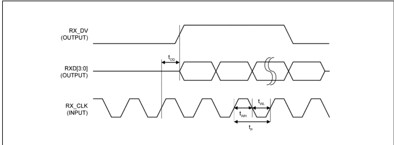
図 6-3: MAC モードの MII 受信タイミング
