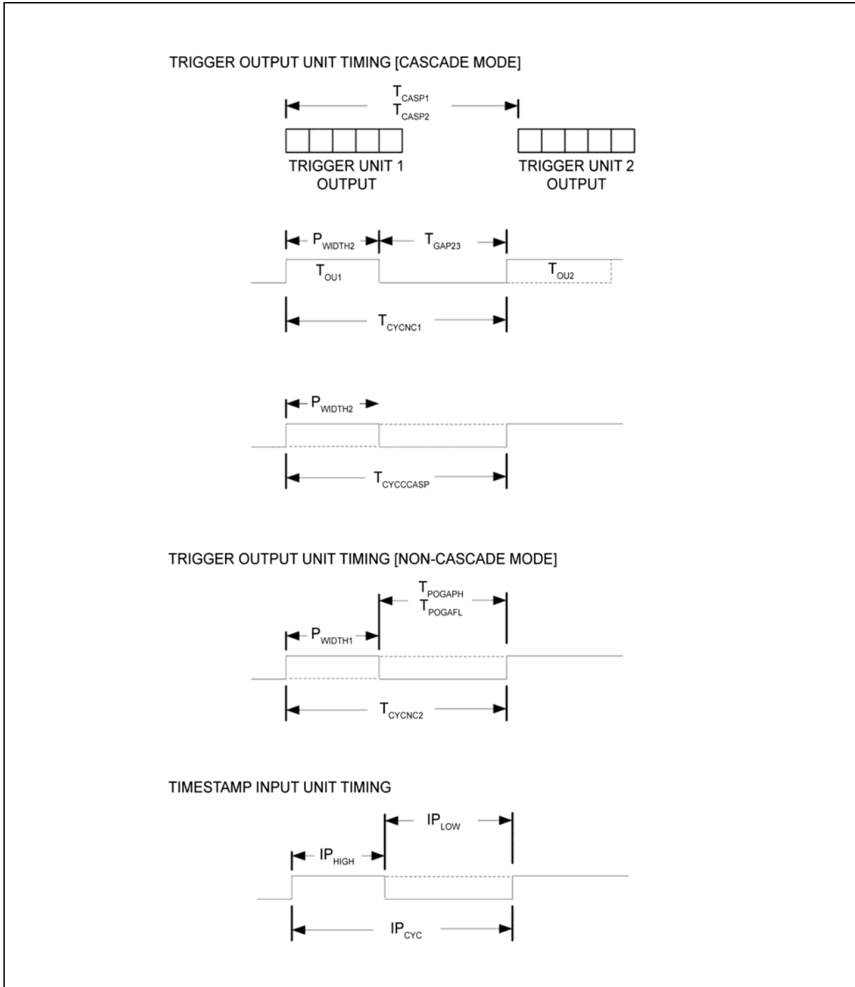
図 6-12: トリガ出カユニットとタイムスタンプ入カユニットのタイミング
