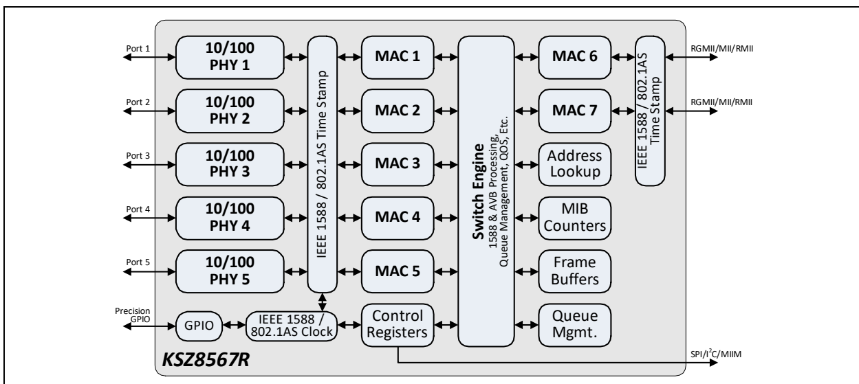
図 2-1: 内部ブロック図
