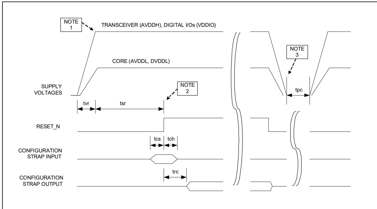
図 6-13: パワーアップおよびリセット タイミング
