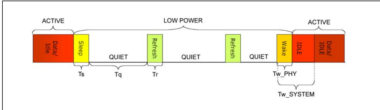
図4-10: トラフィックアクティビティとEEE
