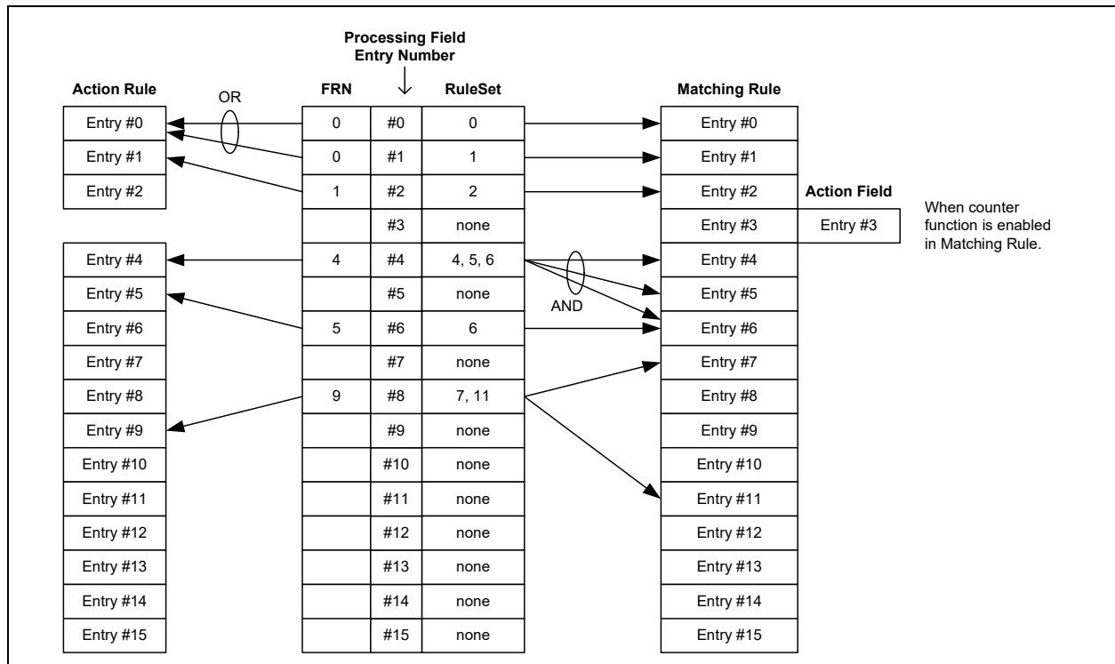
図 4-6: ACL の構造とルール値例
