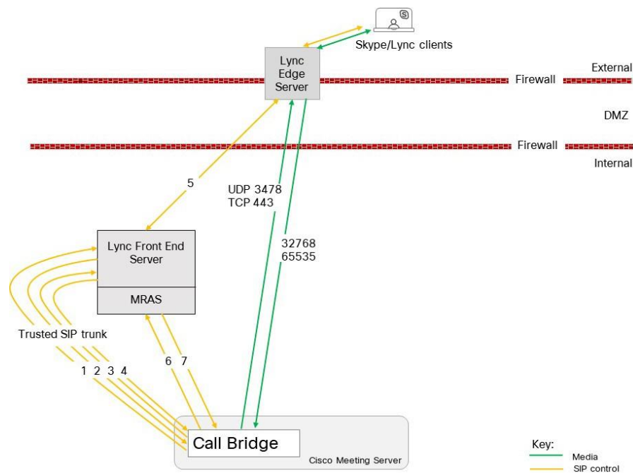
図 37 : Lync Edge サーバーへの Call Bridge のコールフロー
