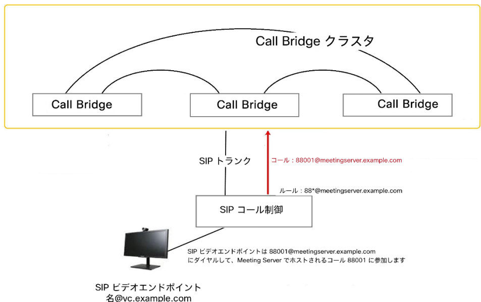
図 33 : Meeting Server でホストされているコールに発信する SIP ビデオエンドポイントの例
