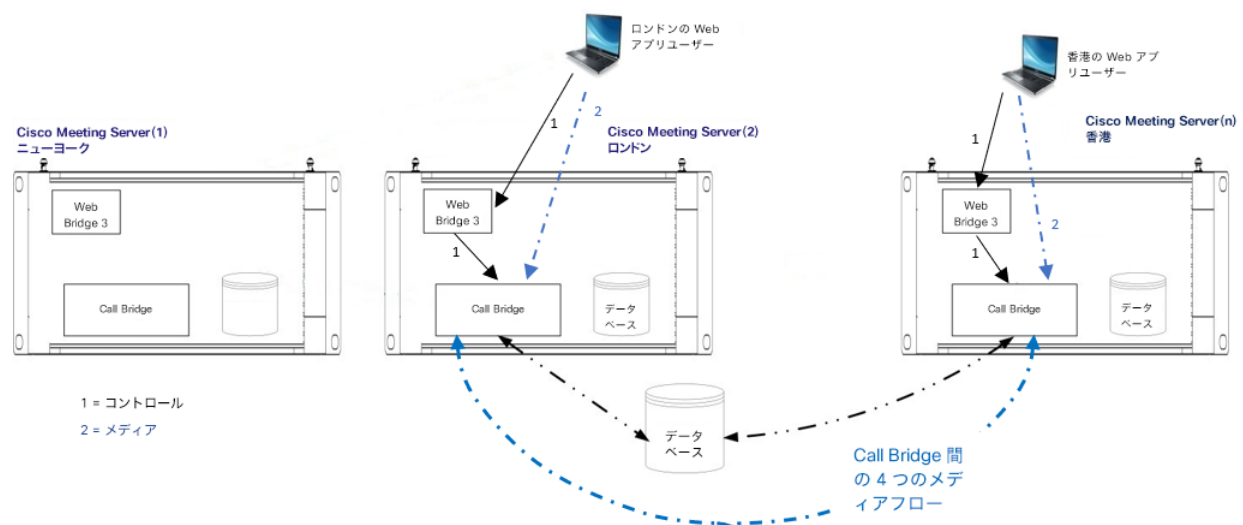
図 27：統合型展開でスペース A にコールする 2 つの Call Bridge
