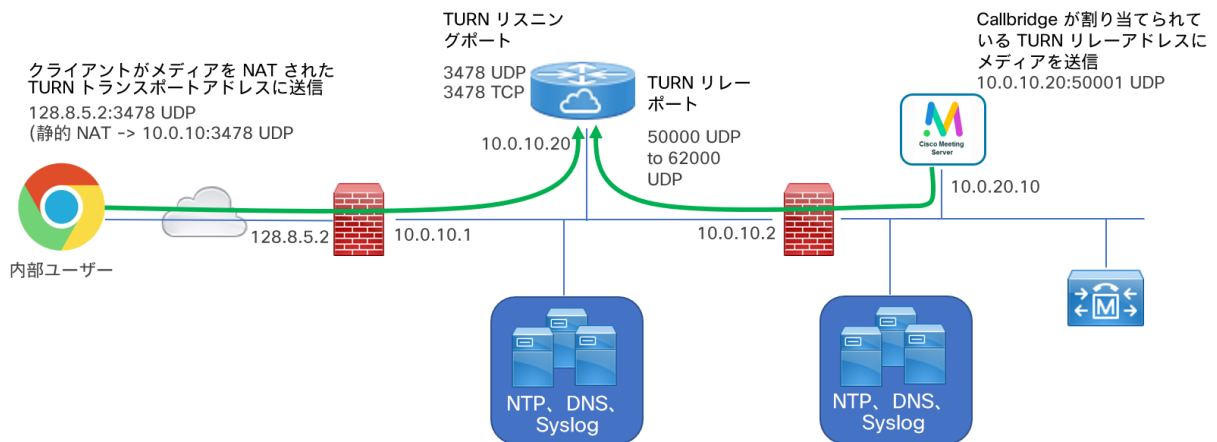
図 13 : UDP を使用した TURN の例
