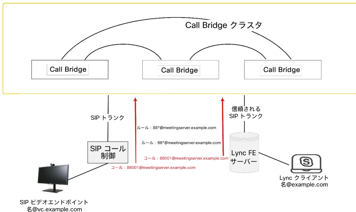
図 35 : Meeting Server でホストされたミーティングに発信する SIP ビデオエンドポイントと Lync クライアントの例
