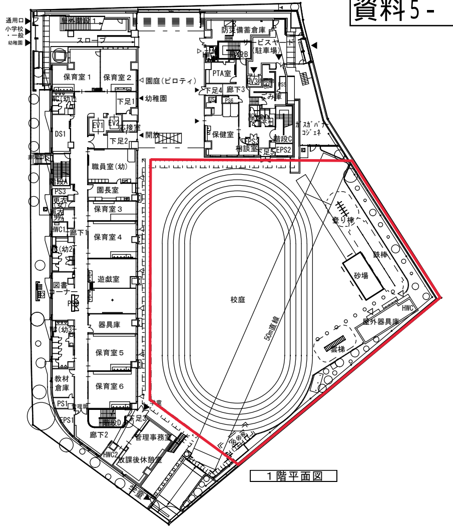
地下1階平面図
