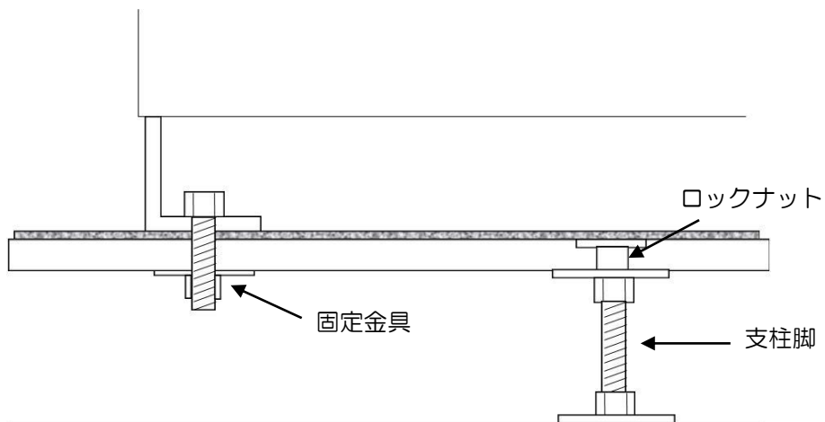
固定された二重床に対する取付け例
