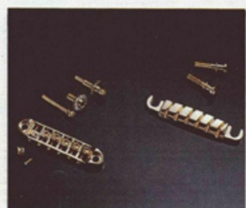
AR全機種に採用のジブラルタル・ブリッジとクイックチェンジ・テールピース
