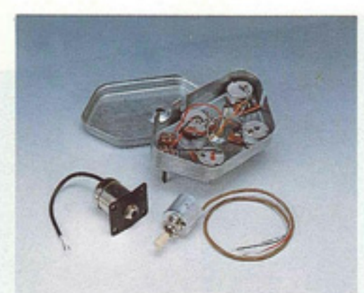
外來ハムノイズをシャット・アウトするシールドング・ボックス (AR300, 305, 550に採用)
