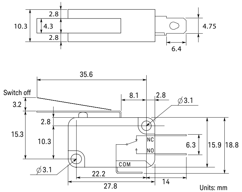
インターロック・スイッチ (N1254A-402) の寸法
