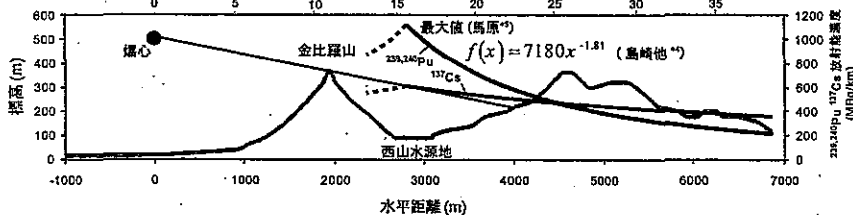
図3. 上の地図上の赤い線は、爆心と金比羅山頂上を通る直線である。下の図の緑の線は、地図上の赤い線を通る地点の爆心からの水平距離と標高をプロットしたもの。下の図で、爆心から金比羅山山頂を通る直線(赤い線)を見ると、西山地区の大部分は、金比羅山によって、爆心からの放射線からさえぎられていたことがわかる。茶色い線は、島崎らによる ^{238,239}\text{Pu} の放射能濃度、紫の線は、同じく ^{137}\text{Cs} の濃度である。馬原による放射能濃度の最大値点は、爆心から2.8 km であるが、そこから西側の地点における放射能濃度については、見積もられていないため、点線で示した。
