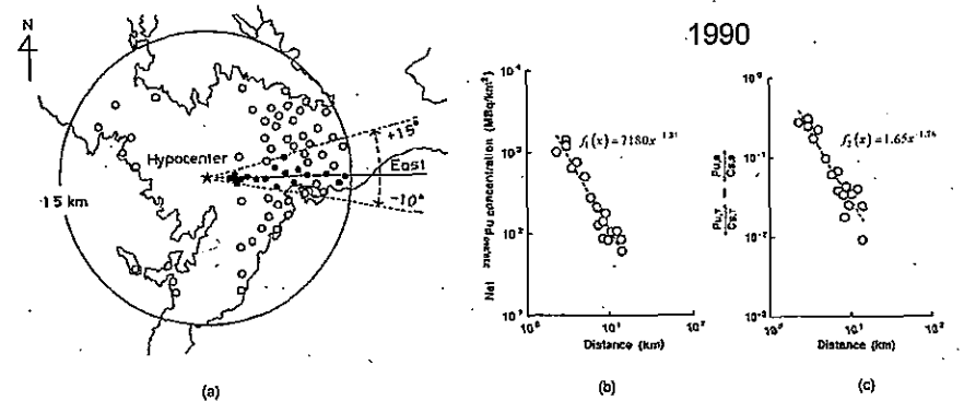
図2. (a) 238,239 Pu試料の採取地。●: 放射能がバックグラウンドより有意に高かったところ。○放射能がバックグラウンドより有意に高くなかったところ。(b) バックグラウンドより有意に高かった地点における距離と 238,239 Puの放射能濃度の関係。(c) 同じく距離と 238,239 Puと 137 Csの放射能濃度の比。放射能濃度は、1990年10月15日現在、バックグラウンド値は爆心地より西側の15地点の平均値を用いた。 f_1 および f_2 は、回帰直線の方程式である。いずれも、島崎他 4) による。
