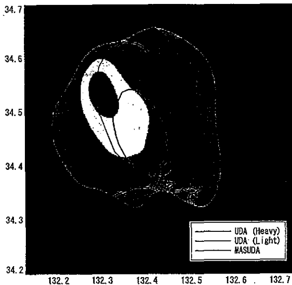
図5. 推定された広島市の黒い雨の降雨時間の地理分布
