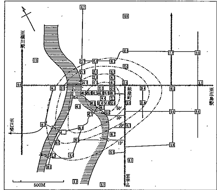
図4. 宮崎らの Neher 型宇宙線計による爆心地周辺の放射線量分布 1945.10.1～10.22.
