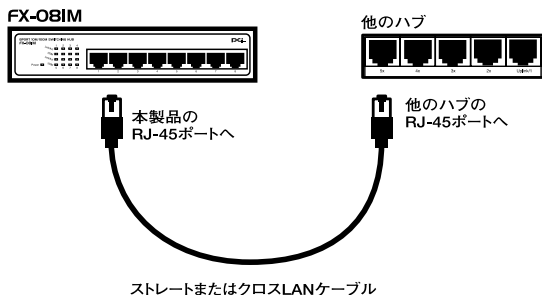
図3-6 カスケード接続図
