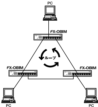
図2-6 ループ図
