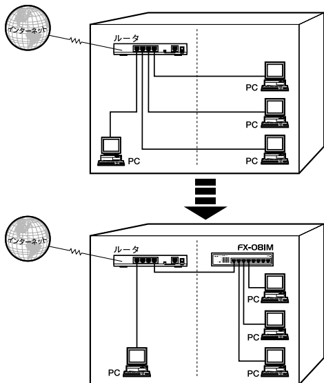
図2-3 複数のケーブルをまとめる
