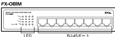
図1-2 前面パネル
