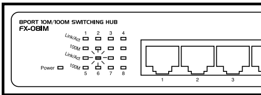
図3-5 Link/Act LED点灯図
