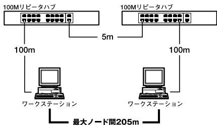
図4-5 100BASE-TXでのカスケード接続の制限
