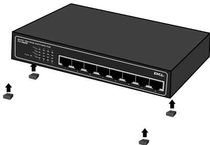
図2-1 ゴム足取り付け図
