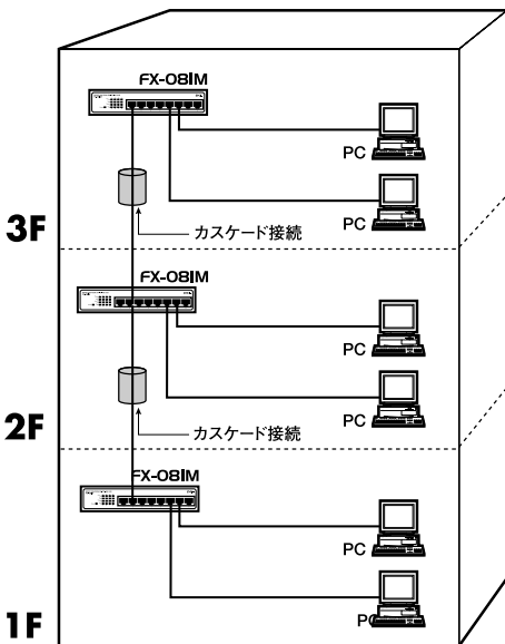
図2-4 各階のカスケード
