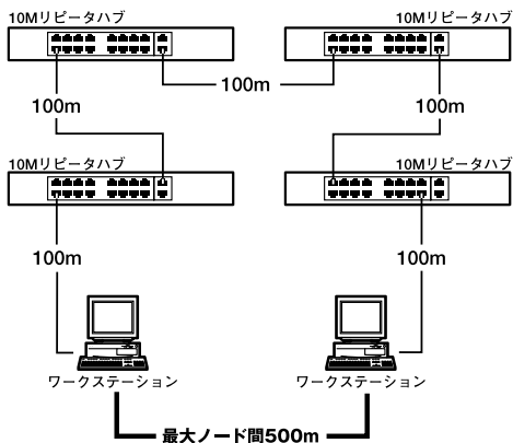
図4-6 10BASE-Tでのカスケード接続の制限
