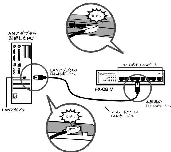
図3-4 コンピュータとの接続図
