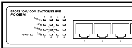
図3-7 カスケード接続時のLink/Act LED点灯図
