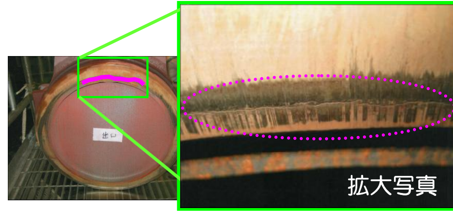
T/D RFP吐出弁(B)シート面のひび
