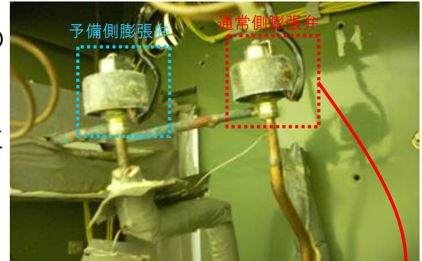
膨張弁（取替前）
