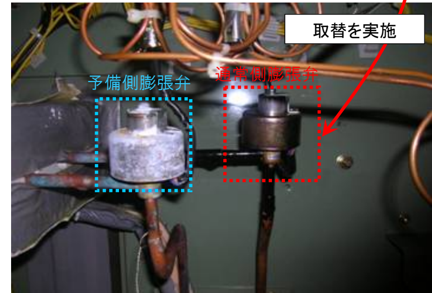
膨張弁（取替後）
