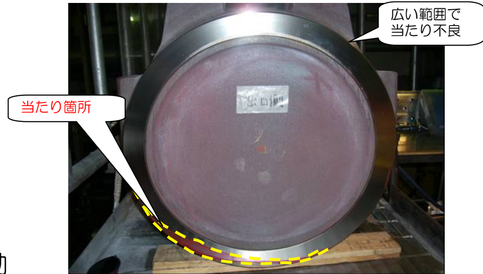
T/D RFP吐出弁 (B) シート面の当たり状況 (手入前)
