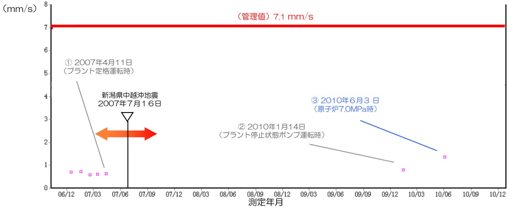
高圧復水ポンプ（B）運転時のカップリング側の振動傾向（水平方向）
