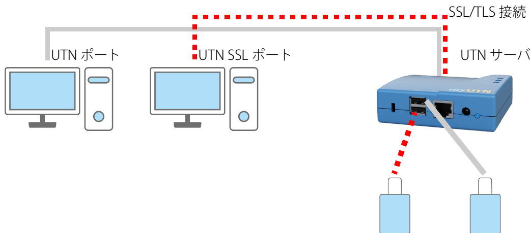
図7： UTN サーバ- ネットワーク内の SSL/TLS 接続
