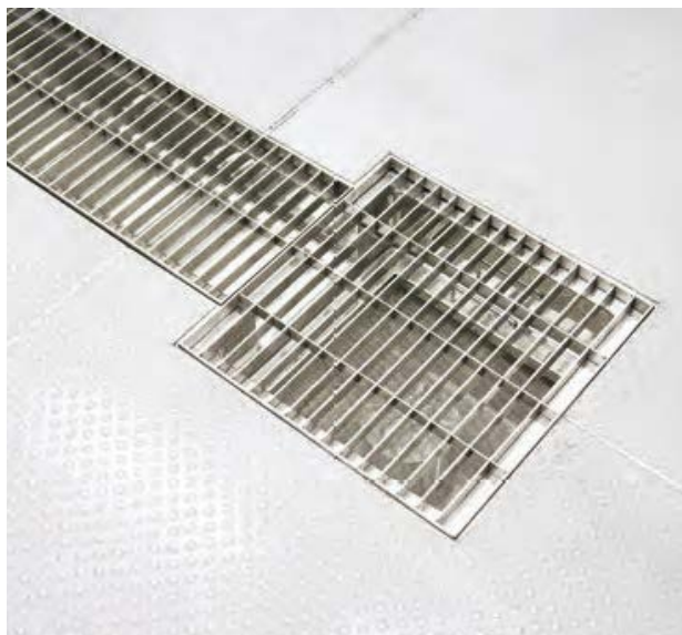
※ポリカプレート、排水柵設置例
