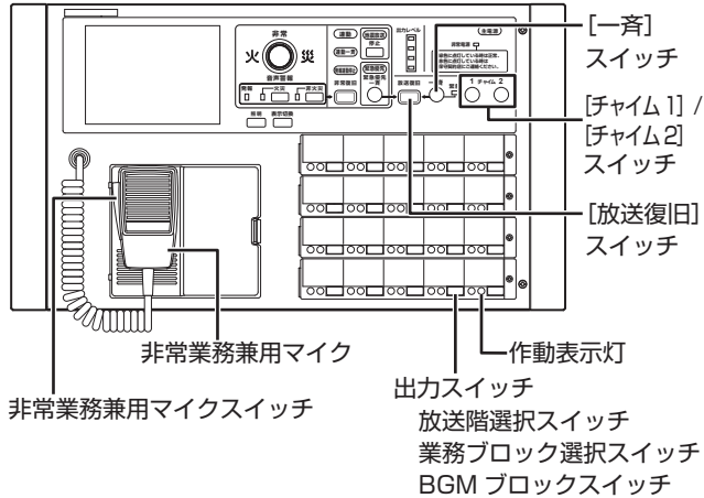
非常業務操作器 (EM-E156)
