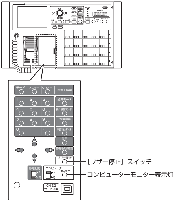
非常業務操作器 (EM-E156)
