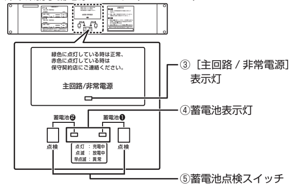
非常業務予備電源ユニット (EM-N152)
