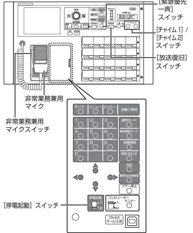
非常業務操作器 (EM-E156)
