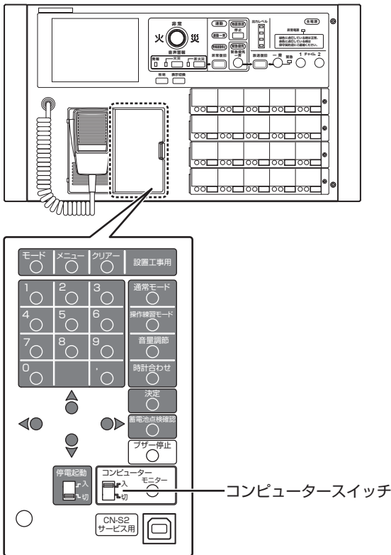
非常業務操作器 (EM-E156)
