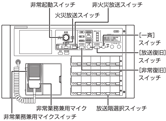
非常業務操作器 (EM-E156)
