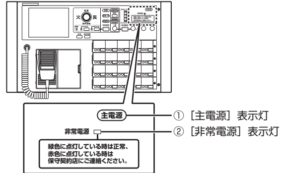
非常業務操作器 (EM-E156)
