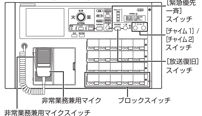
非常業務操作器 (EM-E156)
