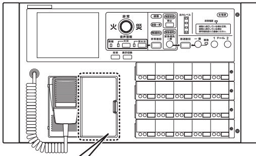
非常業務操作器 (EM-E156)
